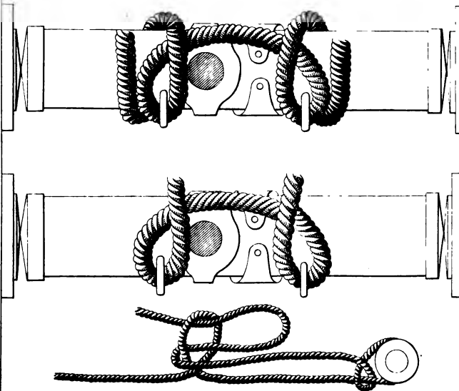
Knot for Manœuvring bolt.
